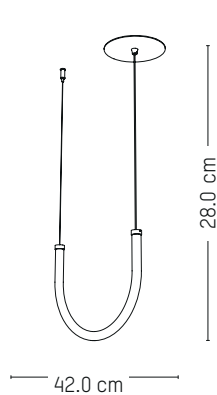
Pendant lamp U
